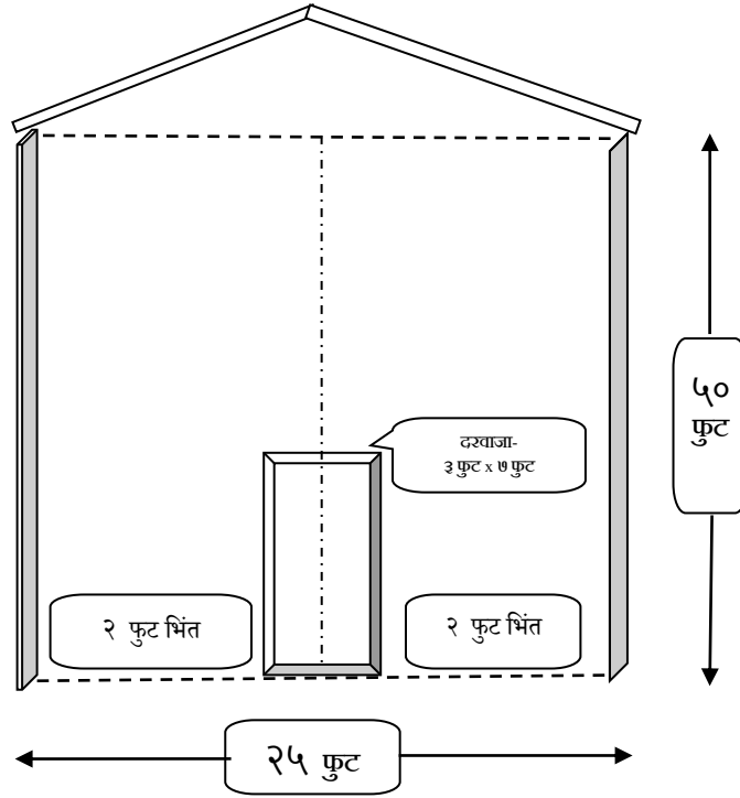
रेशीम किटक संगोपन गृह २५ फुट x ५० फुट
